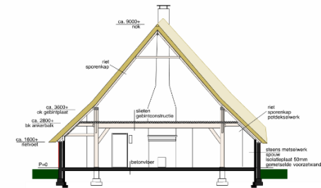
dwarsdoorsnede A-A
